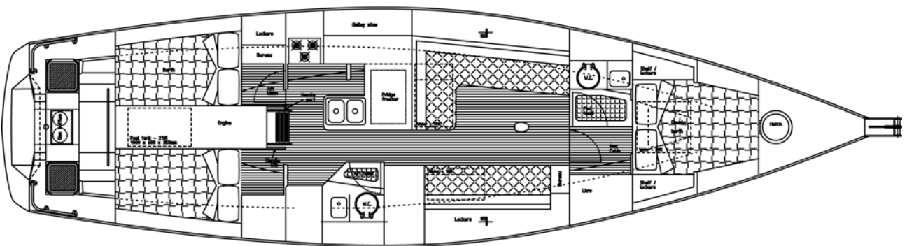
Interiors Plan - Piano degli interni
