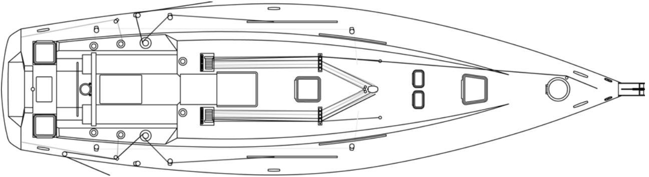
Deck Plan - Piano di coperta
